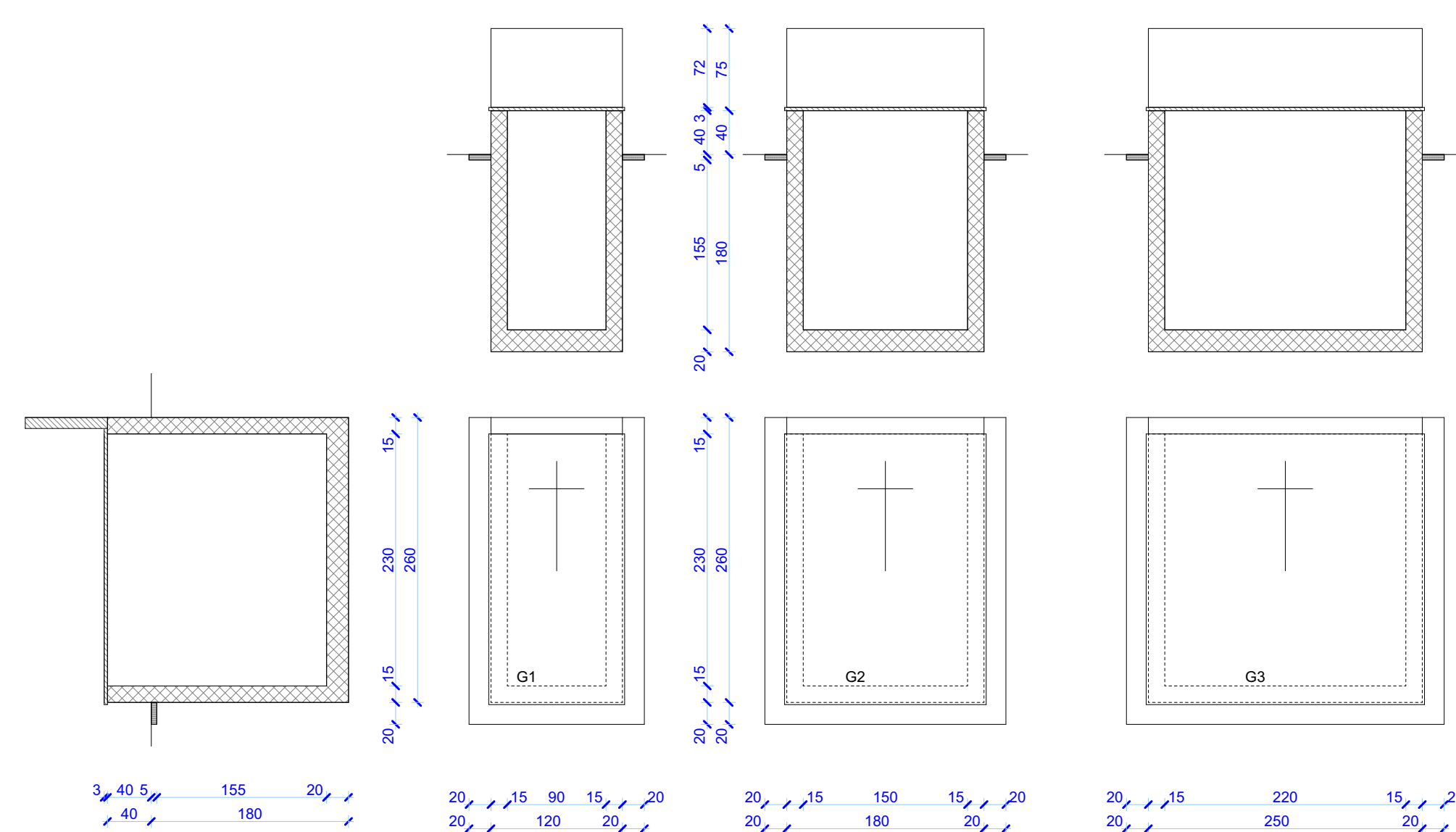
DETALJI GROBNICA MJ 1:50
