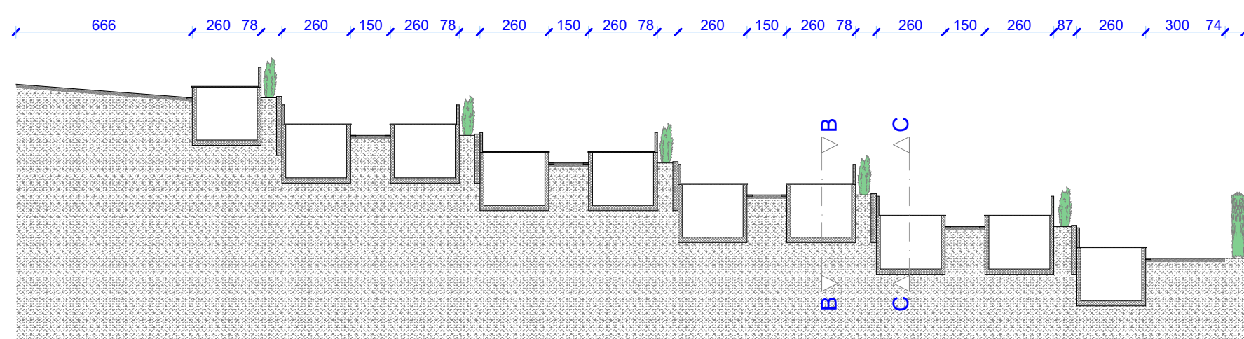
PRESJEK A MJ 1:200
