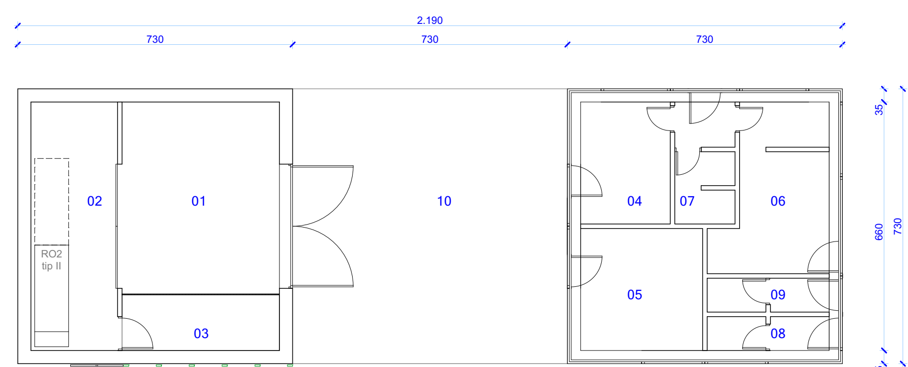
GROBNA KUĆA MJ 1:100
