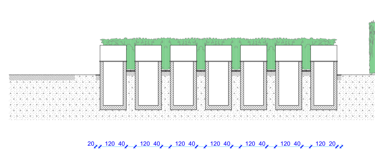
PRESJEK B
