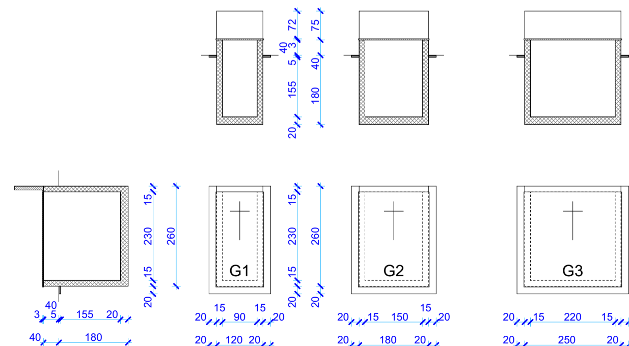
DETALJ GROBNICA MJ 1:50
