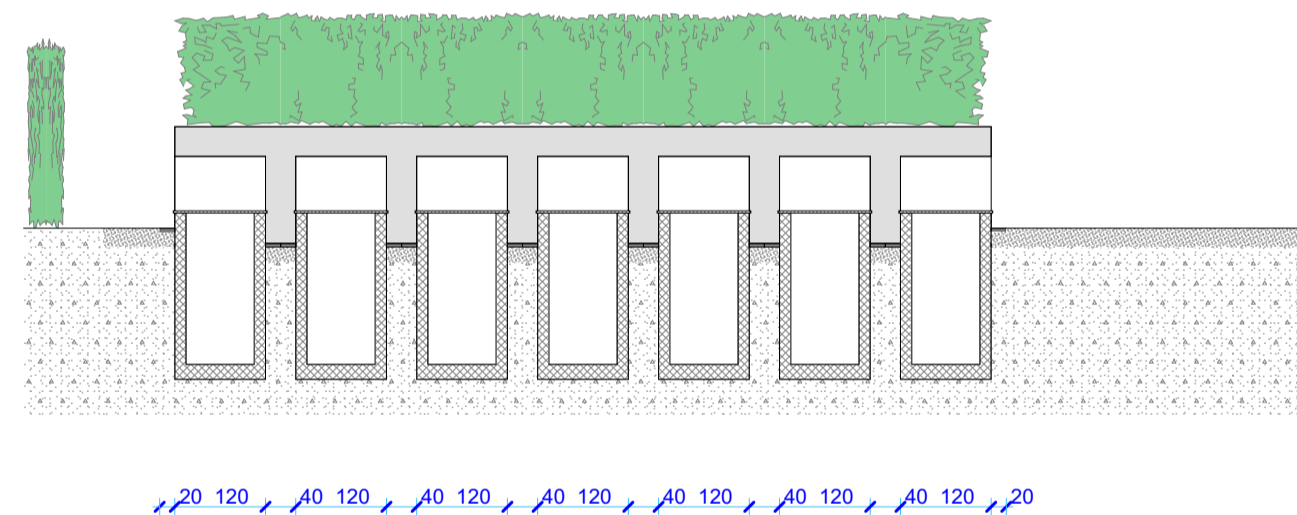
PRESJEK C
